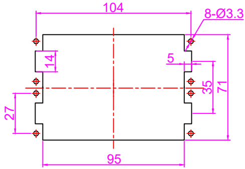
面板开孔图
